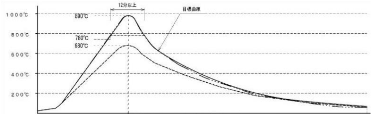
温度 profile 图
